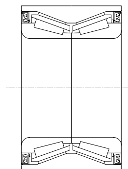
Rodamiento de rodillos cónicos (2 hileras)
