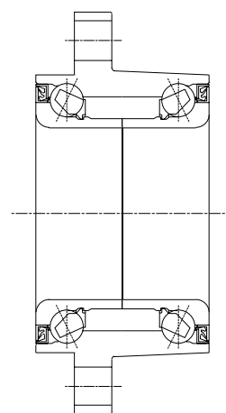
Rodamiento de bolas de contacto angular (2 hileras + 1 brida)
