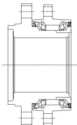
Rodamiento de bolas de contacto angular (2 hileras + 2 bridas)
