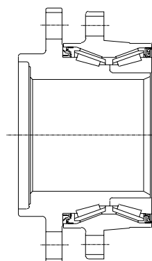
Rodamiento de rodillos cónicos (2 hileras + 2 bridas)
