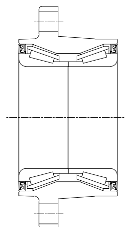
Rodamiento de rodillos cónicos (2 hileras + 1 brida)
