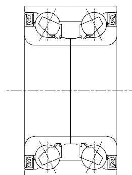
Rodamiento de bolas de contacto angular (2 hileras)
