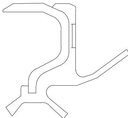
Tres labios de Sellado reforzado
